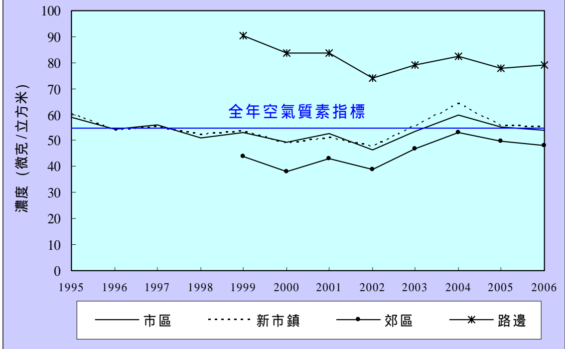
圖 1: 可吸入懸浮粒子(PM10)的長期趨勢
