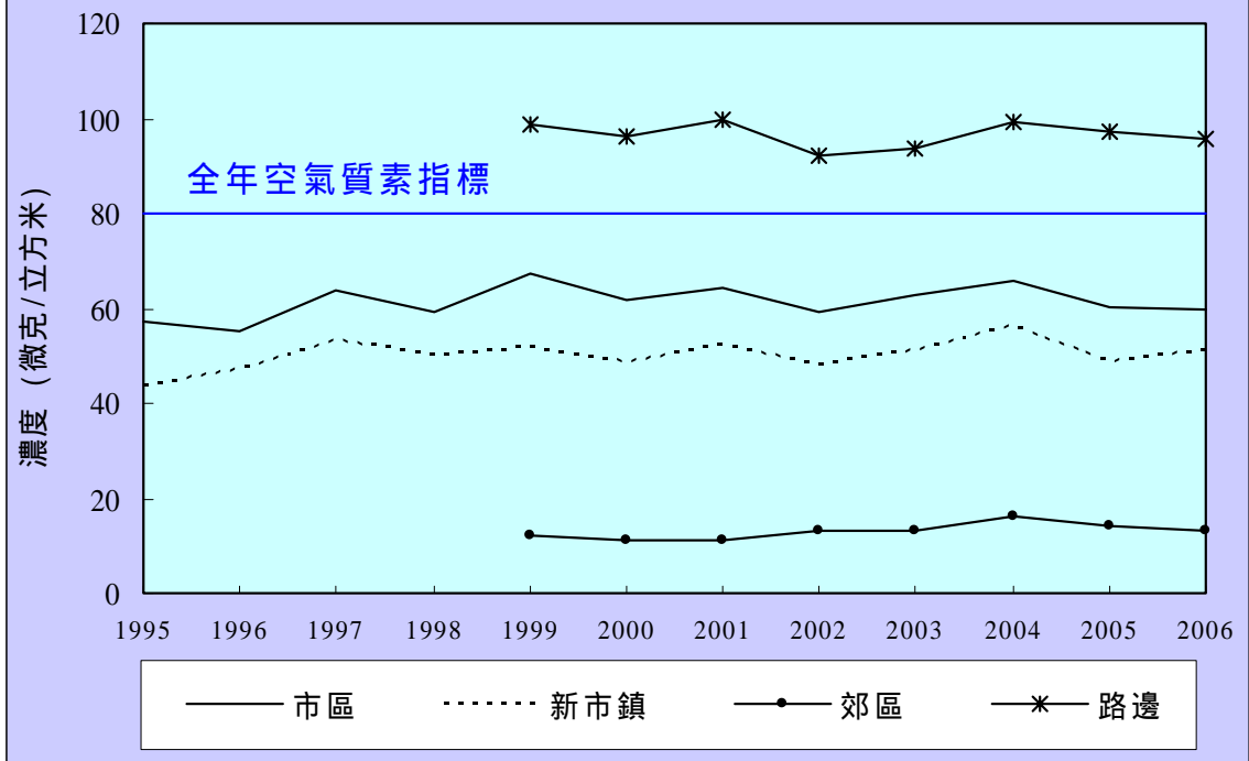
圖 5：二氧化氮(NO 2 )的長期趨勢
