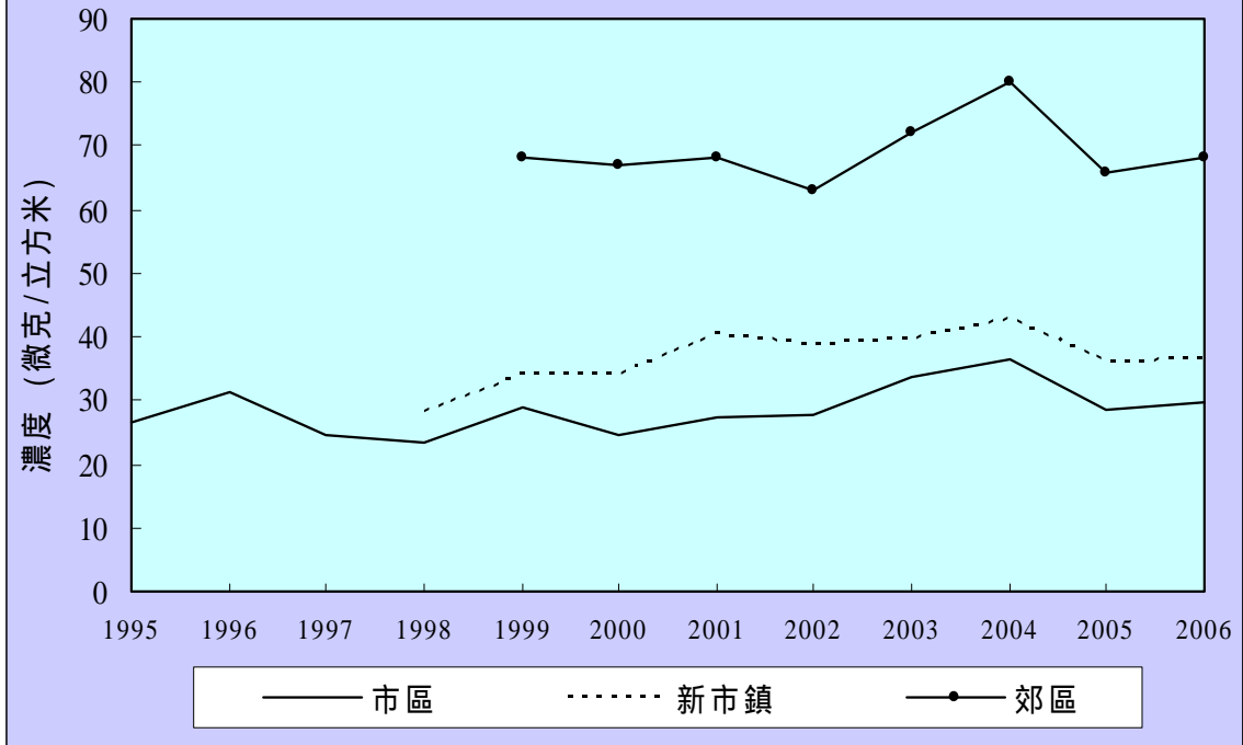
圖 3：臭氧(O 3 )的長期趨勢
