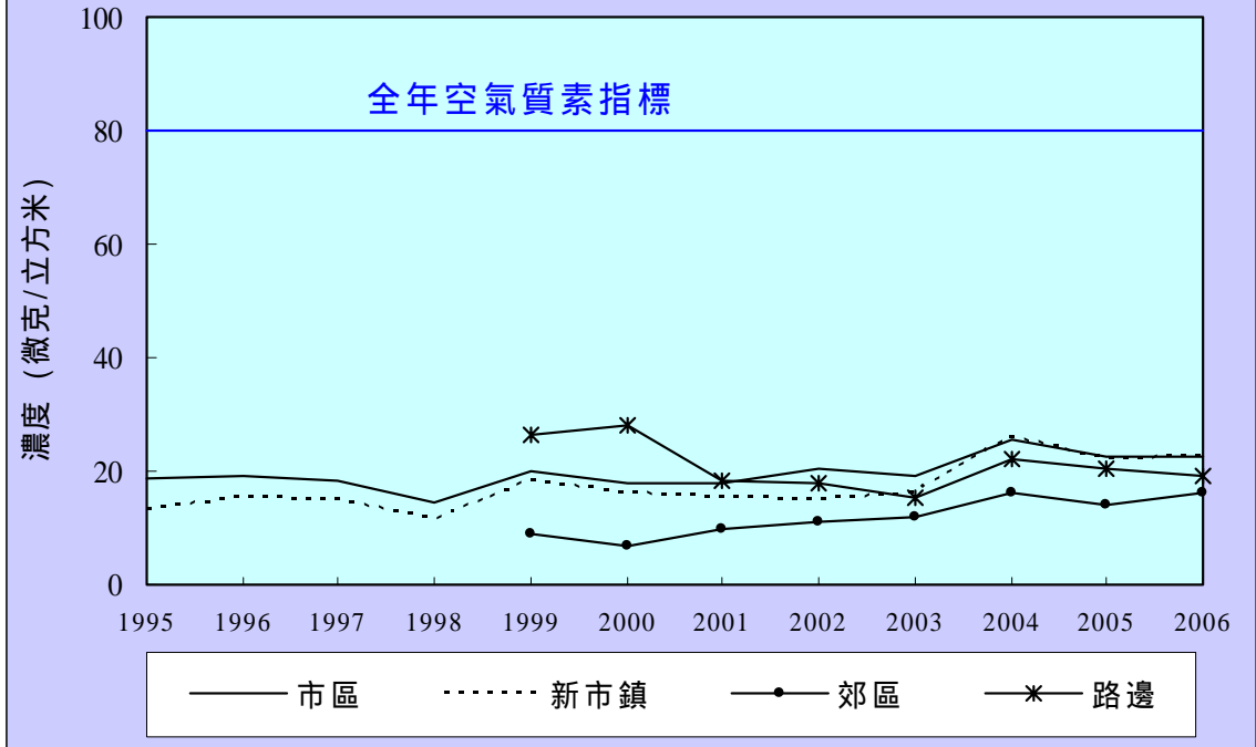
圖 2: 二氧化硫(SO 2 )的長期趨勢
