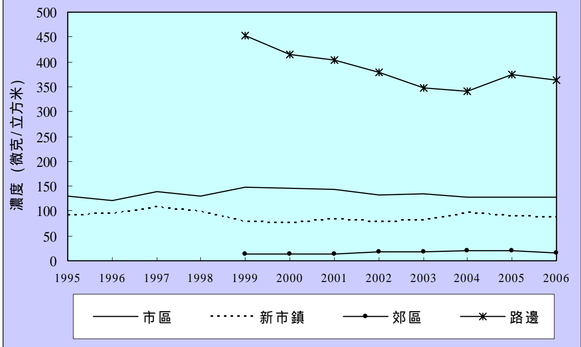
圖 4：氮氧化物(NO x )的長期趨勢
