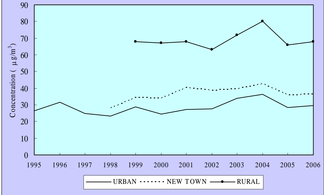
Figure 3 : Ozone (O 3 ) long term trend
